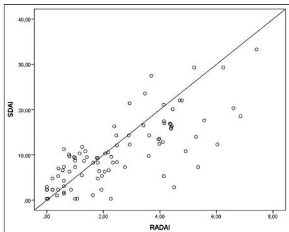
ŞEKİL 3: RADAI ve SDAI değişkenleri arasındaki ilişkiyi gösteren serpmme grafiği.
