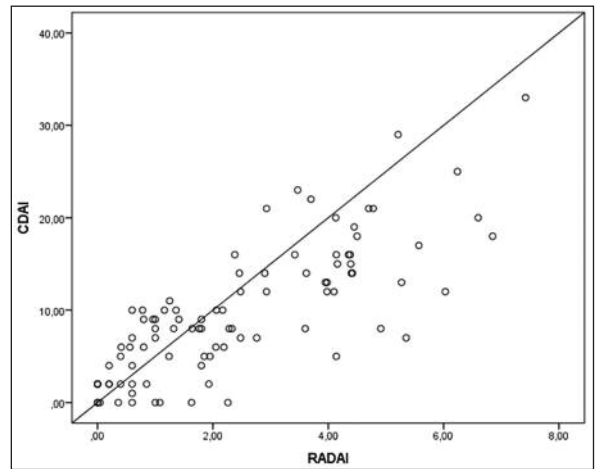
ŞEKİL 2: RADAI ve CDAI değişkenleri arasındaki ilişkiyi gösteren serpmme grafiği.
