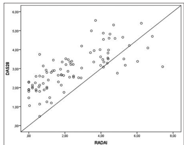
ŞEKİL 4: RADAI ve DAS28 değişkenleri arasındaki ilişkiyi gösteren serpmme grafiği.
