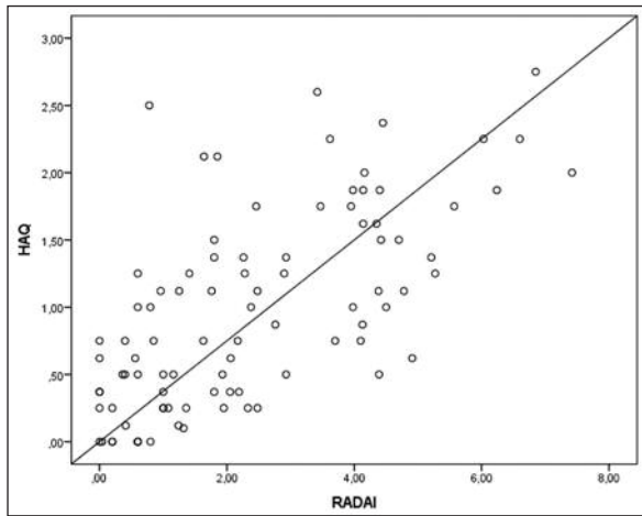
ŞEKİL 1: RADAI ve HAQ değişkenleri arasındaki ilişkiyi gösteren serpmme grafiği.
